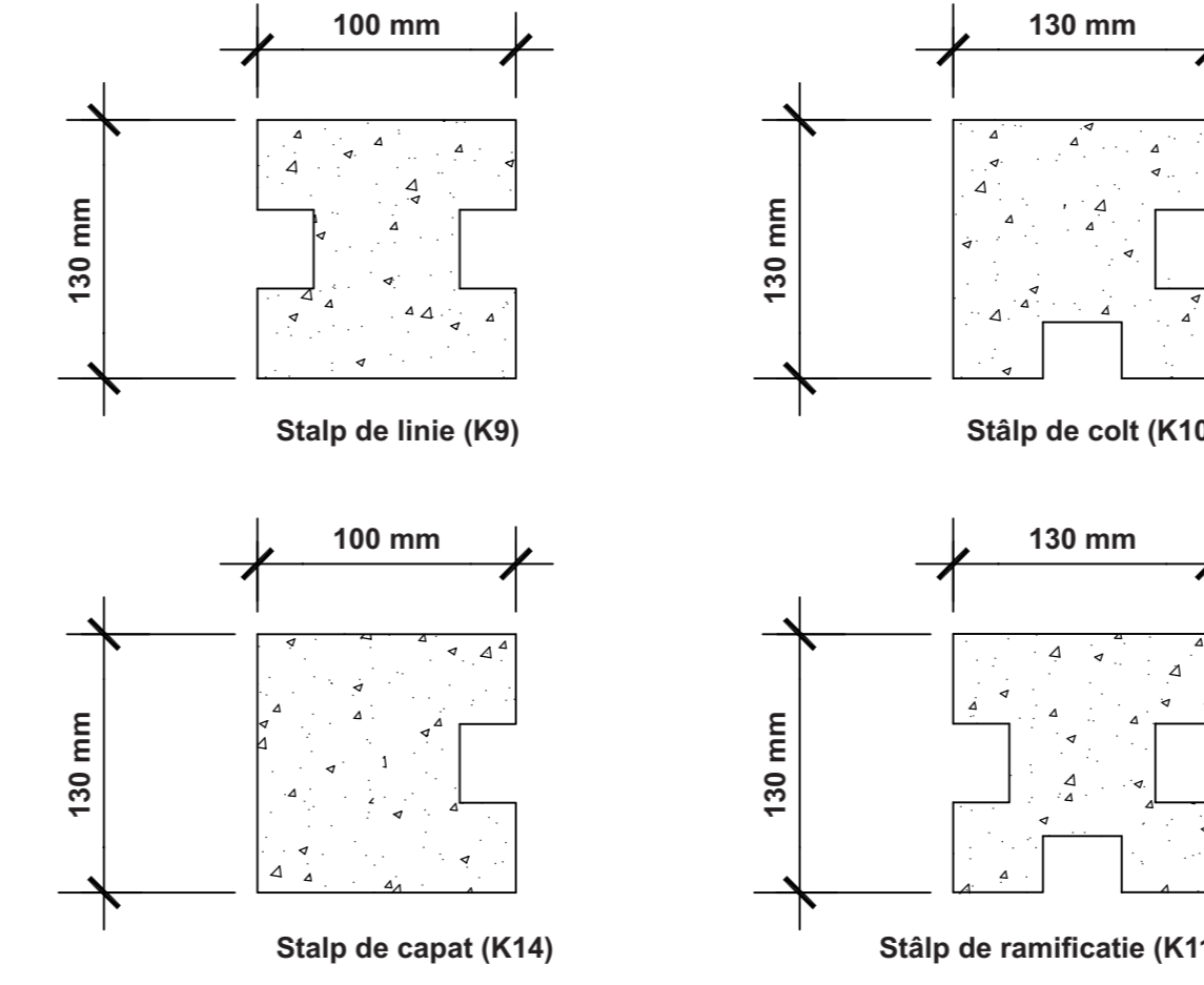
SECTIUNE STALP GARD
